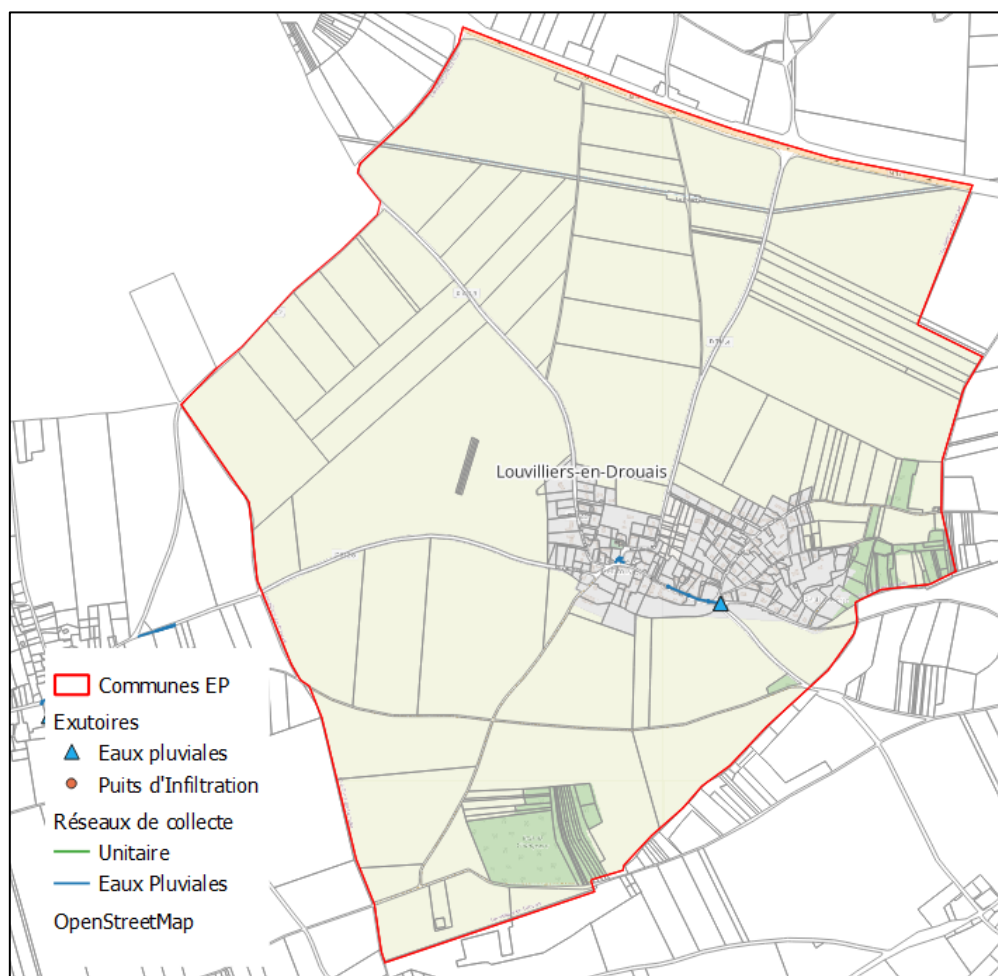
Figure 2 Plan des réseaux sur la commune de Louvilliers-en-Drouais
